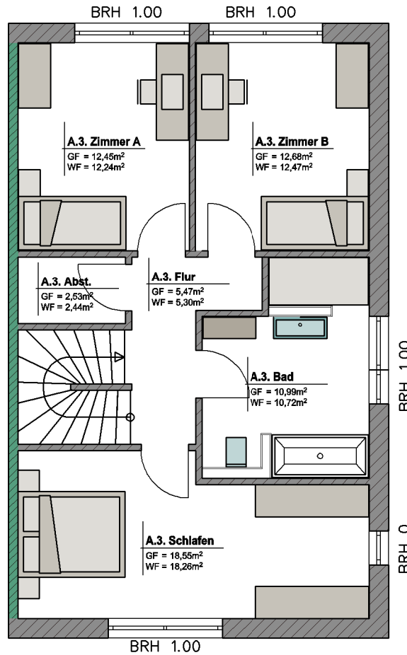
Obergeschoss
