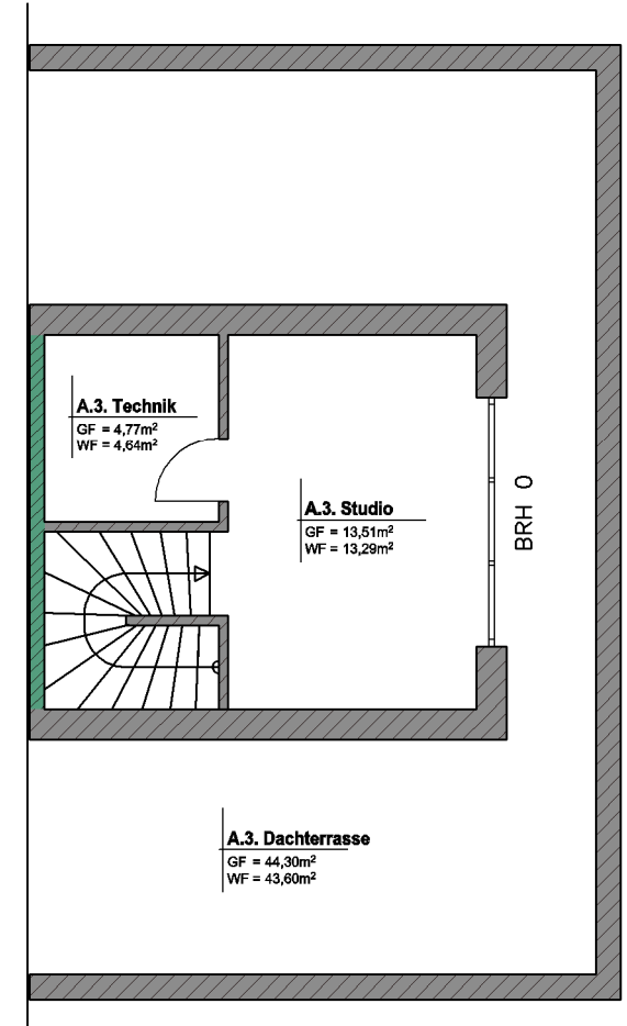
Dachgeschoss
